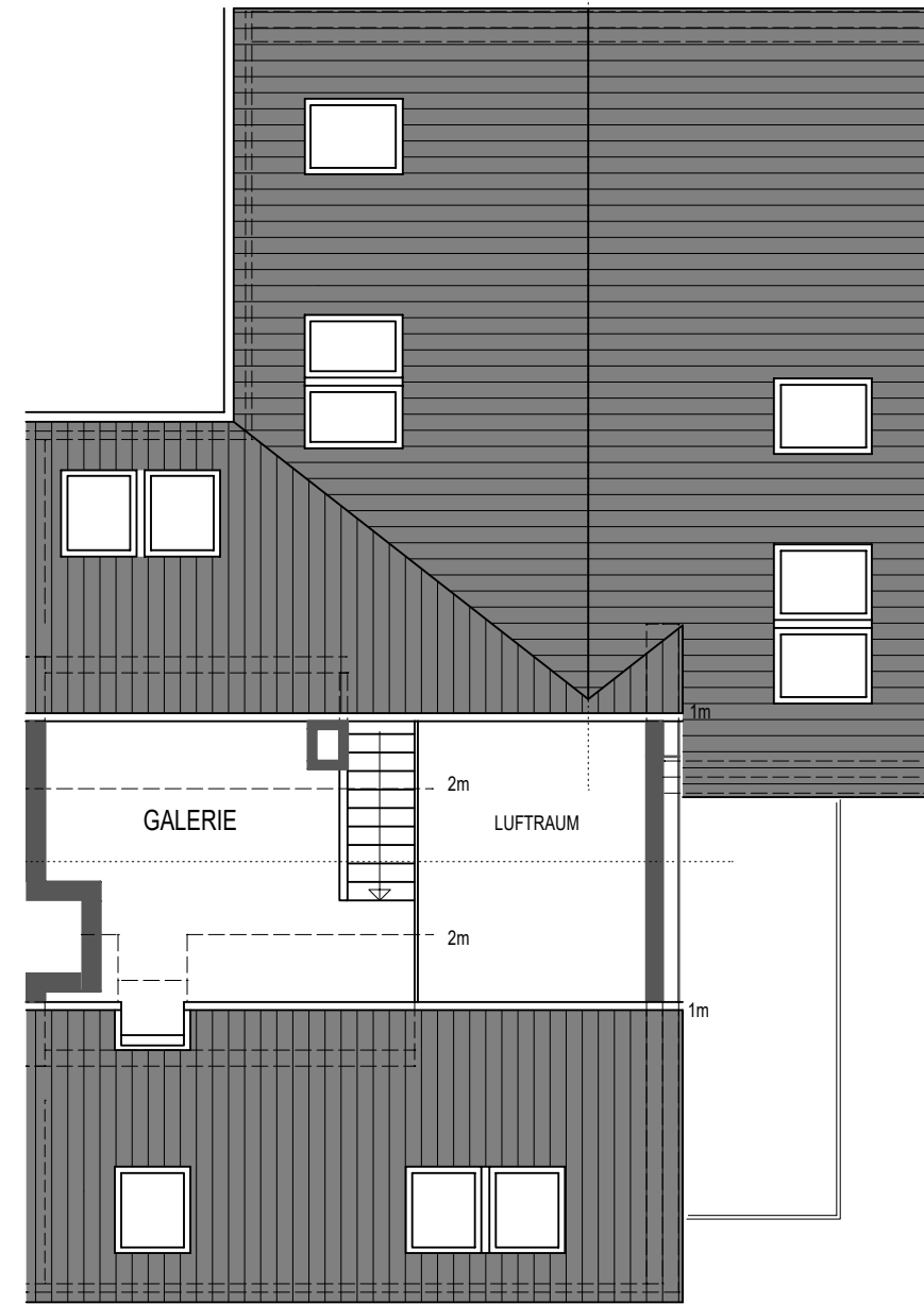
2.DACHGESCHOSS
