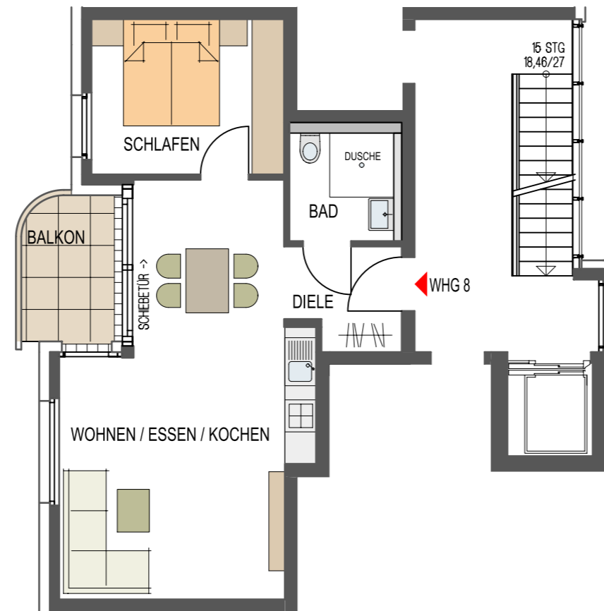
2.OBERGESCHOSS MAßSTAB : 1 - 100
