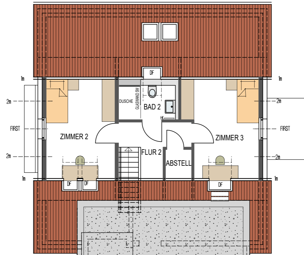
2.DACHGESCHOSS MAßSTAB : 1 - 100
