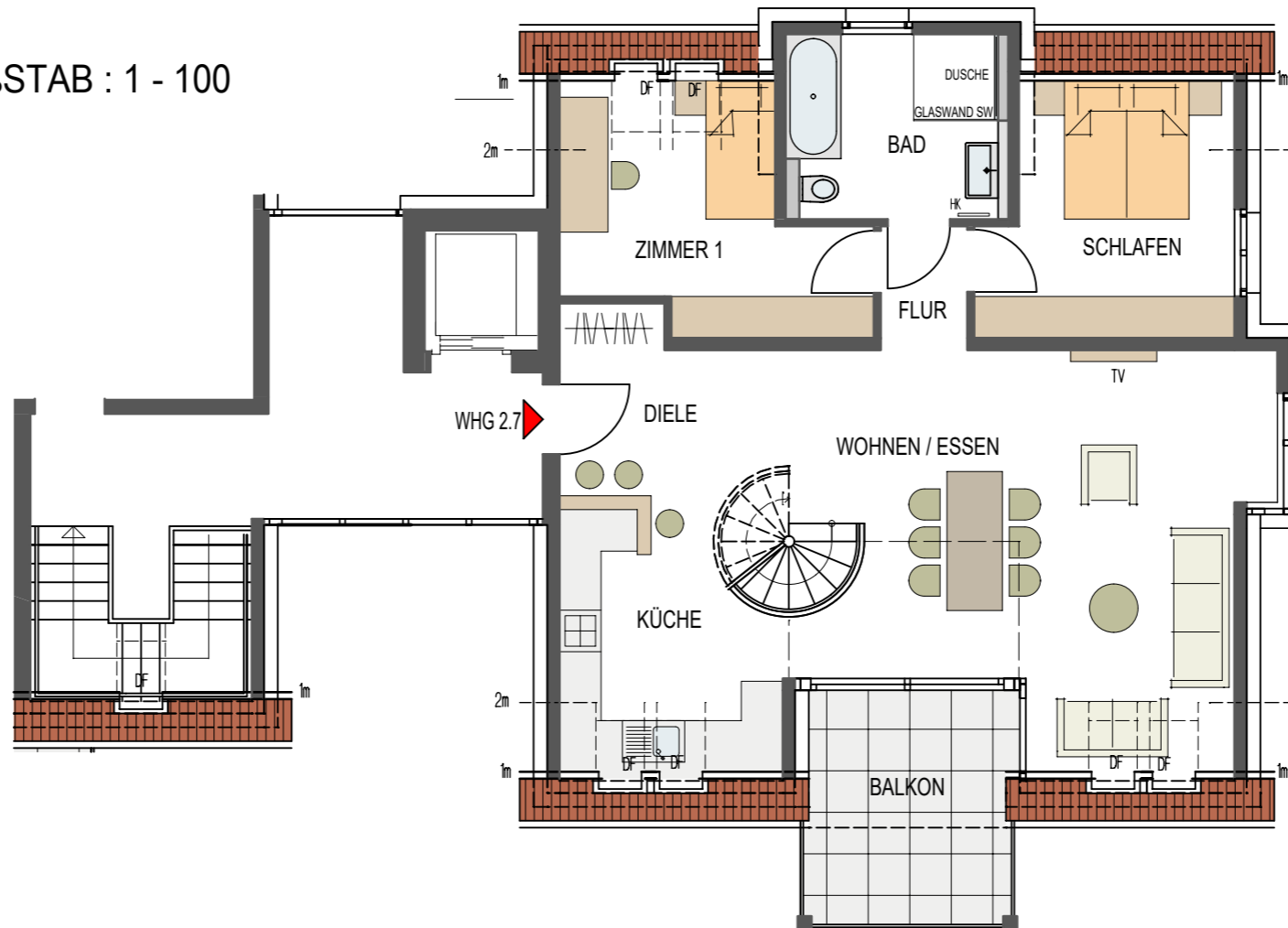
1.DACHGESCHOSS MAßSTAB : 1 - 100
